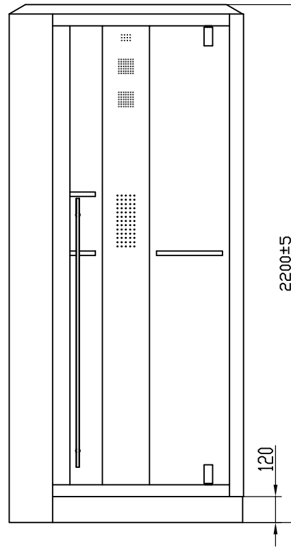
SR-89101RS 线框图 1000*1000*2200 (mm)
